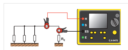
Metodo con 2 pinze – Schema di principio
