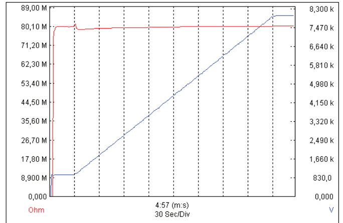
MODULO MEG Grafico delle prove V(t), R(t) sulla resistenza di isolamento fissa
