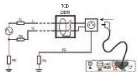
Esempio: prova RCD tramite presa a muro in un sistema TT.
